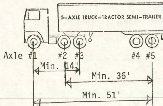
5-Axle TTST
