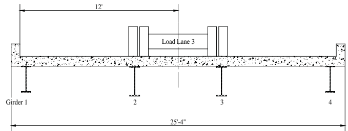
a. Lane 3 Loading
