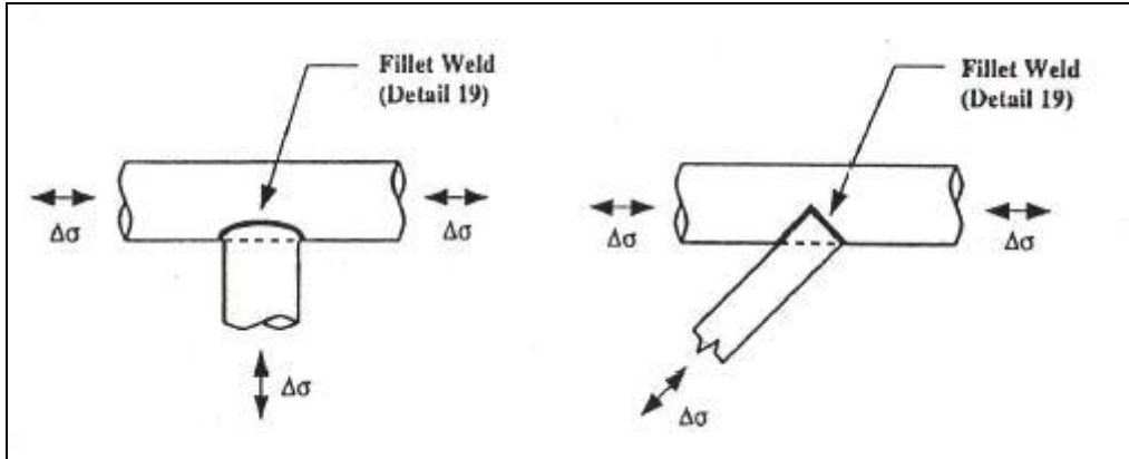
Fig. 60 ET stress category (AASHTO, 2010)
